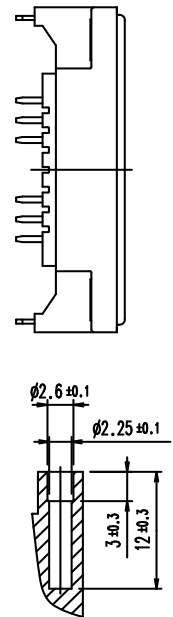
Section A-A
